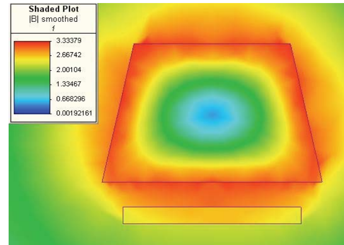
Inward taper
